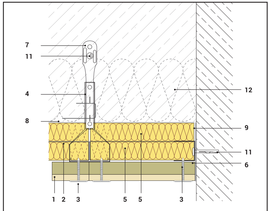
ANSICHT FRONTAL
