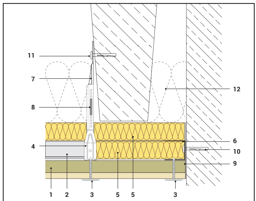
ANSICHT SEITLICH
